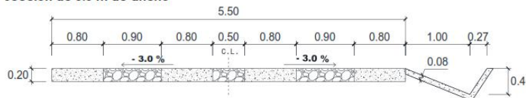
Sección de 5.5 m de ancho
