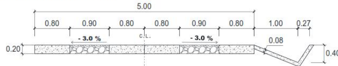
Sección de 5.0 m de ancho
