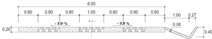
Sección de 6.0 m de ancho
